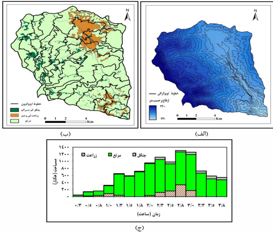
شکل ۲- نقشه توپوگرافی حوزه آبخیز گلاز (الف)، نقشه پراکنش کاربری اراضی و موقعیت خطوط هم‌زمان تمرکز (ب) نحوه توزیع کاربری‌ها در بخش‌های مختلف هیستوگرام زمان- مساحت حوزه آبخیز گلاز (ج)
