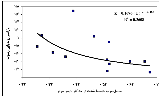
شکل ۳- ارتباط بین پارامتر روندیابی رسوب با حاصل‌ضرب شدت بارندگی موثر در بیشینه بارش موثر در حوزه آبخیز گلاز، آذربایجان غربی
