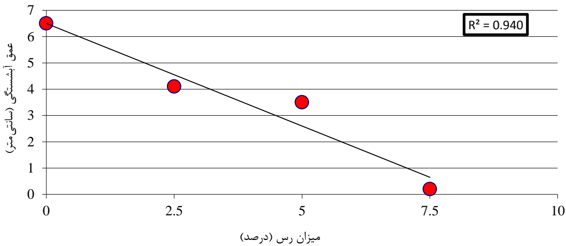
شکل ۶- عمق آبشستگی در ابتدای دیواره
