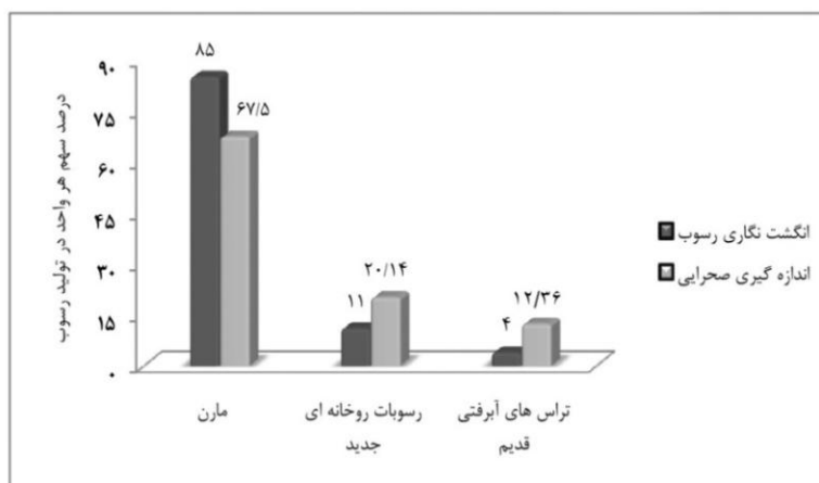
شکل ۷- بررسی میزان تطابق سهم‌های واحدهای سنگ‌شناسی در تولید رسوب به دو روش انگشت‌نگاری رسوب و اندازه‌گیری مستقیم صحرایی در حوزه آبخیز ایده‌لو
