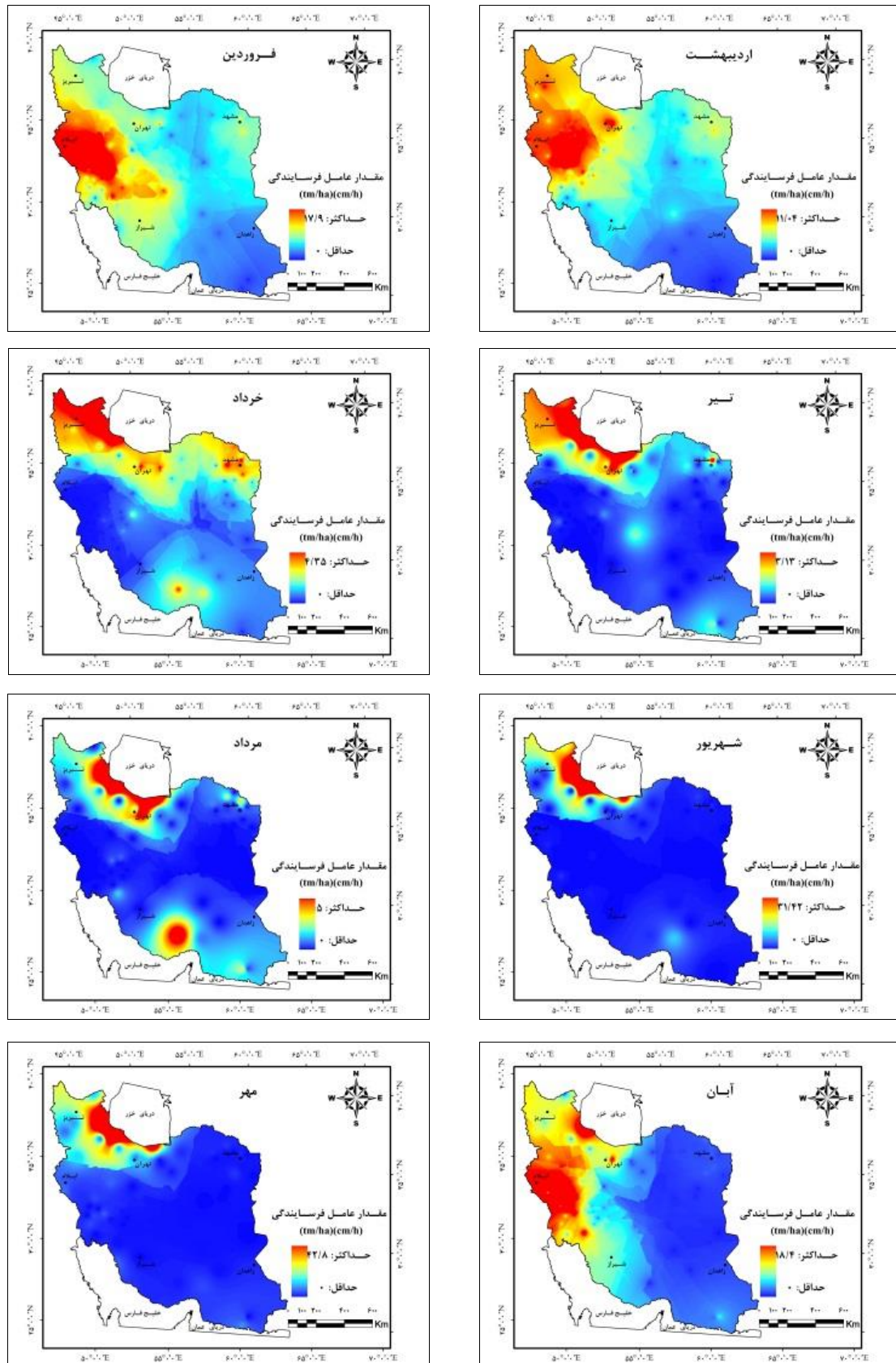
شکل ۲- نقشه‌های عامل فرسایشی باران در مقاطع زمانی مختلف در ایران
