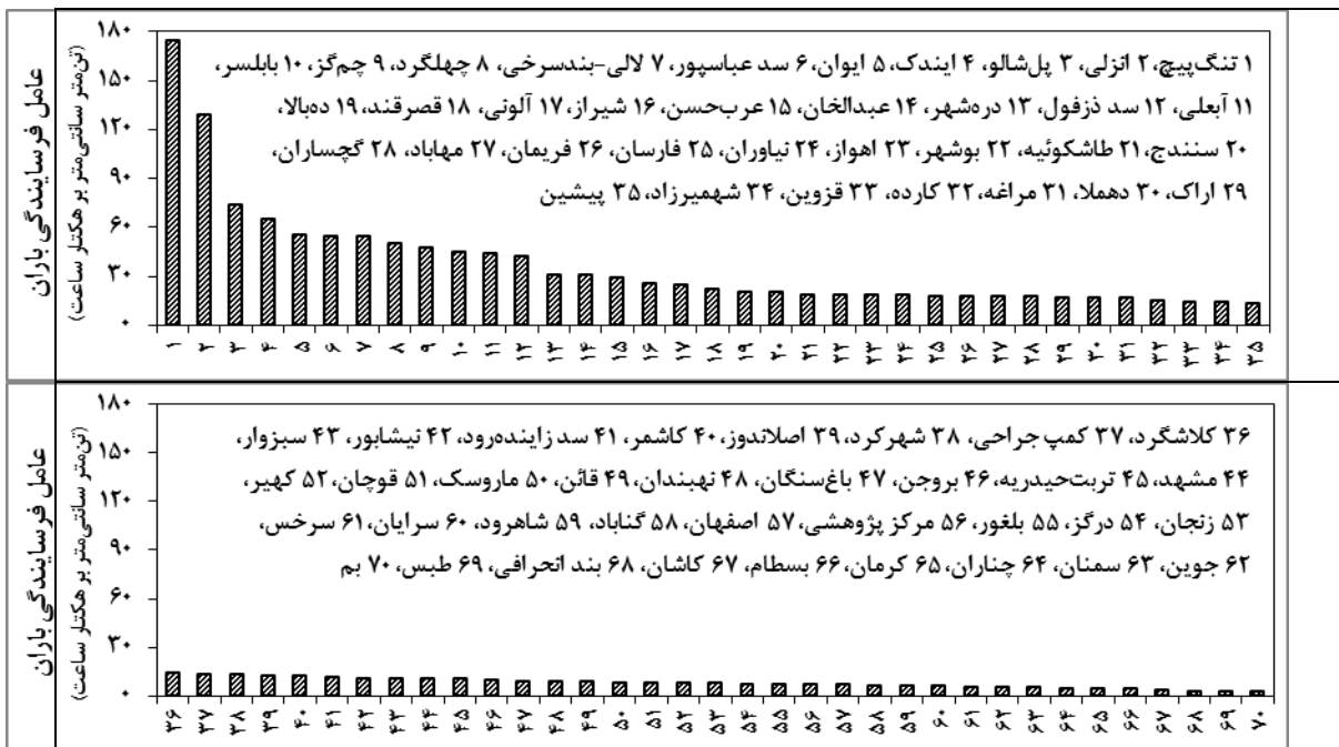
شکل ۳- اولویت‌بندی خطر عامل فرساینده‌گی باران سالانه در ایستگاه‌های مطالعاتی در کشور
