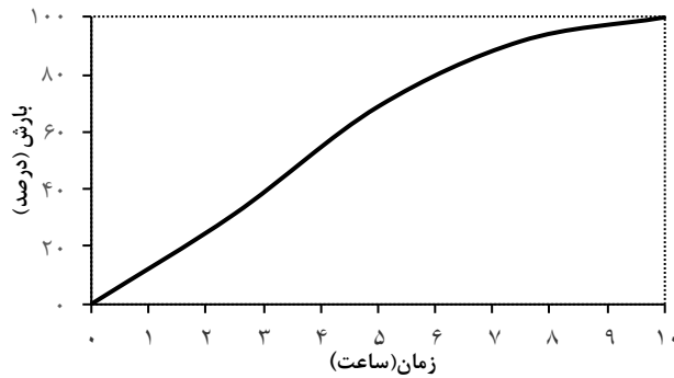
شکل ۵- منحنی معرف توزیع زمانی بارش ۱۰ ساعته حوزه آبخیز خانمیرزا
