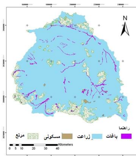
شکل ۳- نقشه کاربری فعلی اراضی حوزه آبخیز تلوارمهرآباد
