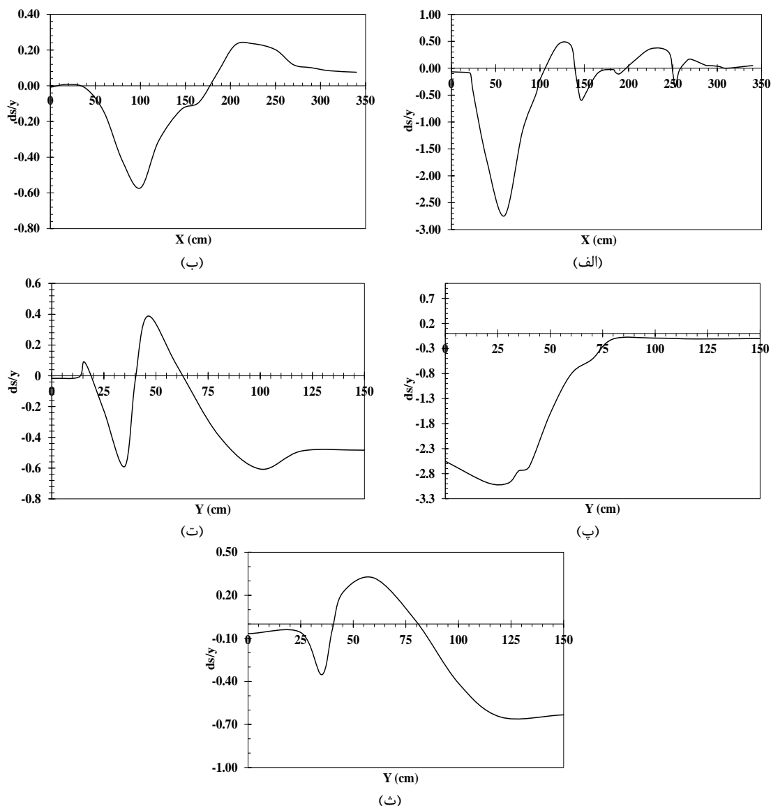
شکل ۷- عمق بی بعد آبشستگی برای ترکیب T6 (L T T)، الف) مقطع طولی در محل نوک آبشکن‌ها، ب) مقطع طولی در وسط کانال، پ) مقطع عرضی در محل نوک دماغه آبشکن اول، ت) مقطع عرضی در محل نوک دماغه آبشکن دوم و ث) مقطع عرضی در محل نوک دماغه آبشکن سوم
