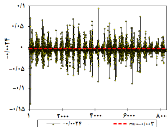
شکل ۱۵- نمودار آزمون جابه‌جایی سیگنال خطا
